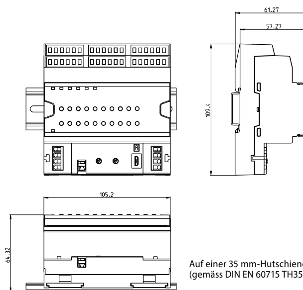
Gehäuse mit 6 TE (105 mm) Passend für Elektroschaltschrank (gemäss DIN 43880, Grösse 2 x 55 mm)
