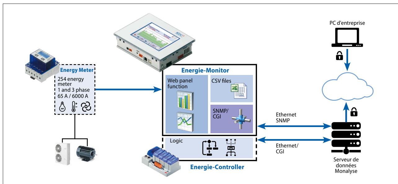
▲ Principe de fonctionnement d'une analyse d'exploitation avec E-Monitor et Monalyse
