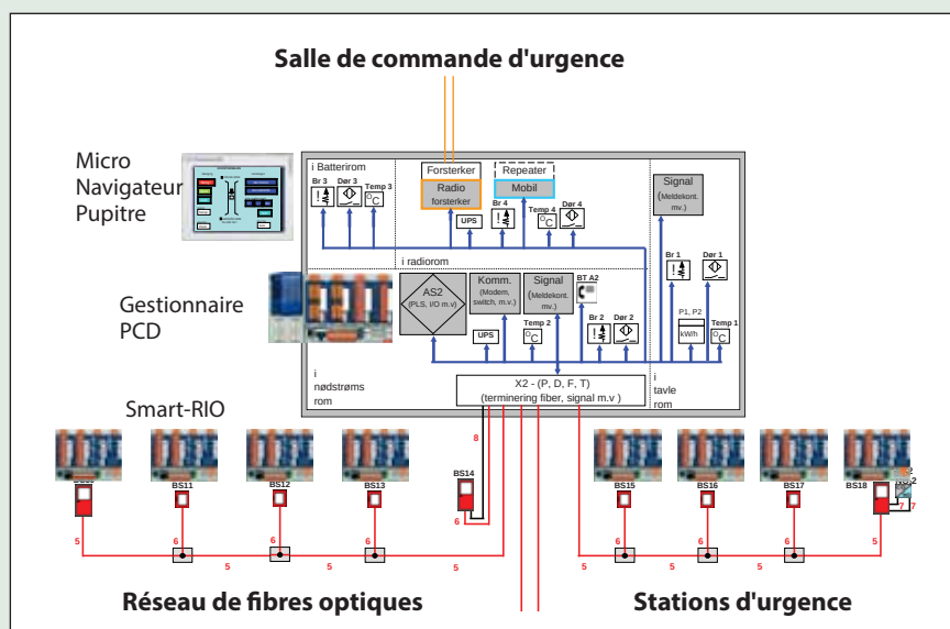
▲ Plus de 80 Smart RIO Saia® PCD3.T665 sont utilisés dans les stations d'urgence pour la surveillance du téléphone, des extincteurs etc.
