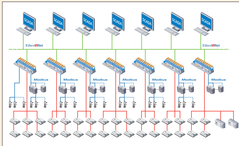
▲ Le système d'automatisation de Bustaffa après réparation suite au dégât des eaux. La transformation a été achevée sans interruption de la production. Le système SCADA n'a pas du être modifié.
