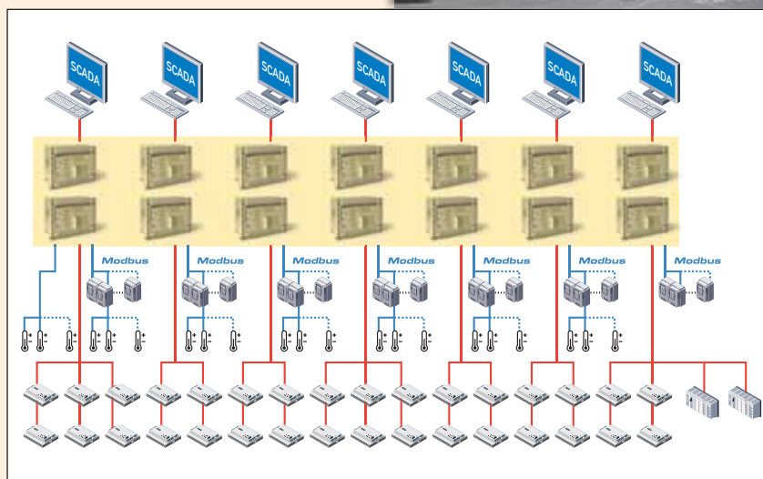
▲ Le système d'automatisation de Bustaffa datant de 20 ans – les Saia® PCD6 représentés en jaune – ont dû être remplacés en raison d'un dégât des eaux.
