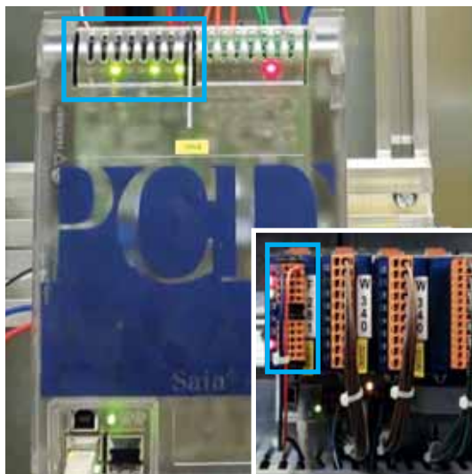
▲ Modules de communication et E/S conventionnelles combinées : Saia® PCD1.M2120 avec M-Bus et PCD3.M3330 avec Belimo MP-BUS
