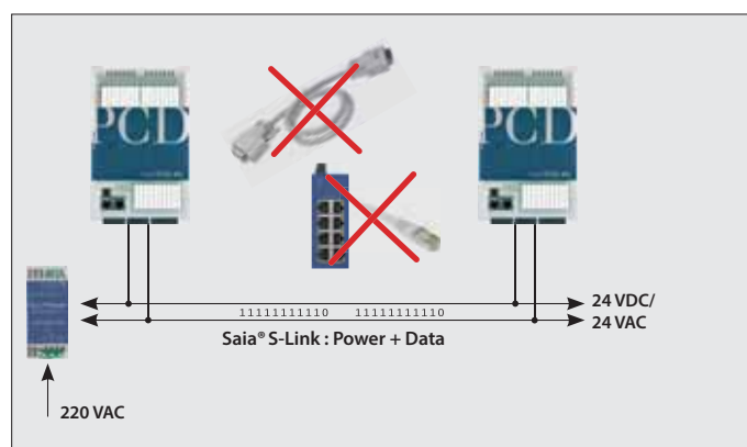
▲ Diagramme de principe « Saia-S-Link » : structure du système avec Saia® PCD1. La communication s'effectue sans raccord de câbles spécialisé.
