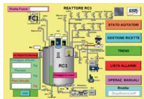
▲ Capture d'écran de l'IHM WEB pour le réacteur chimique, créé avec Saia® WebEditor 5.14
