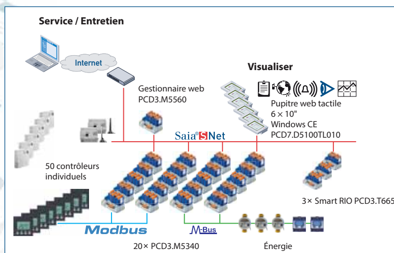
▲ Topologie de réseau de la technique du bâtiment chez MarcCain. Unité centrale performante Saia®PCD3.M5560 avec serveur d'automatisation comme station centrale de gestion pour l'exploitation et l'entretien
