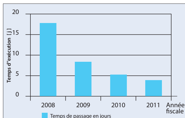
L'effet Lean : temps de passage en jours – du lancement de la production jusqu'à l'emballage, exemple des « compteurs d'énergie ».
