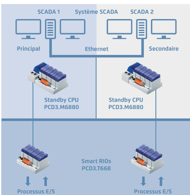
Réseau physique partagé dans une topologie en étoile avec des composants standard
